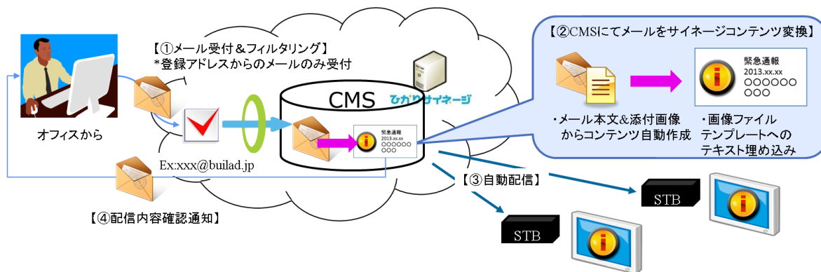
図3 「スピードメッセージ」機能イメージ図
