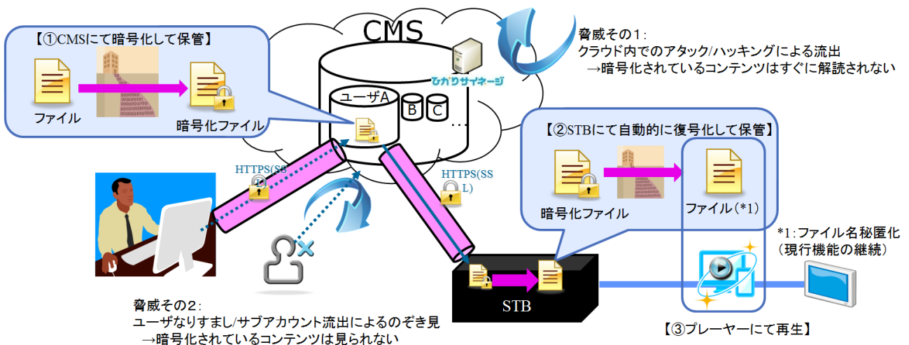
図2 「暗号化」機能イメージ図
