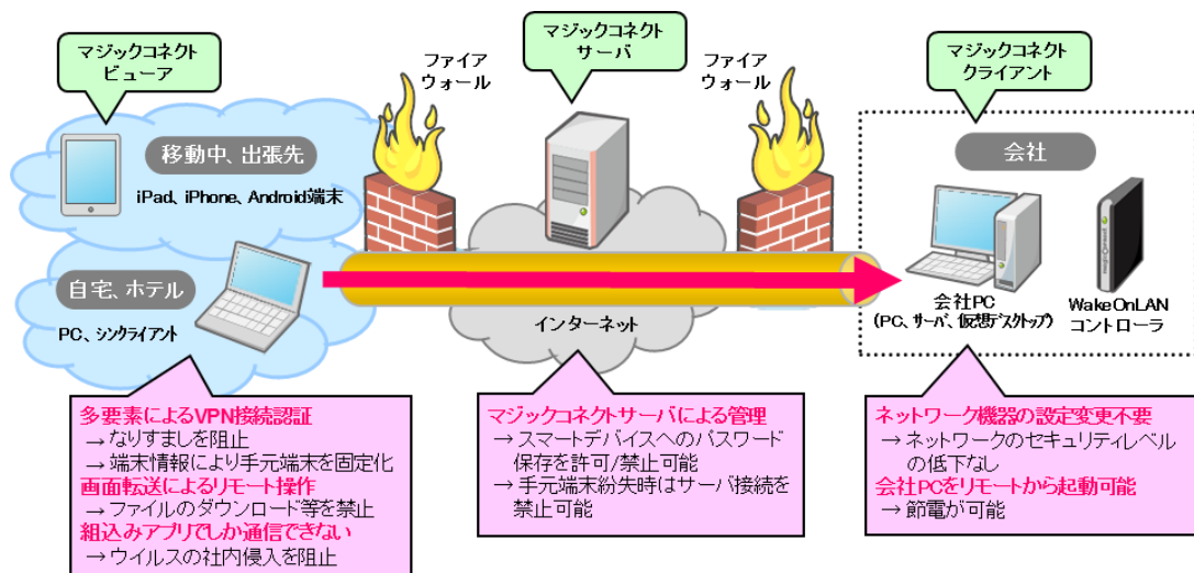
図1 マルチデバイス対応の端末認証型「マジックコネクト」クラウドサービスの構成
