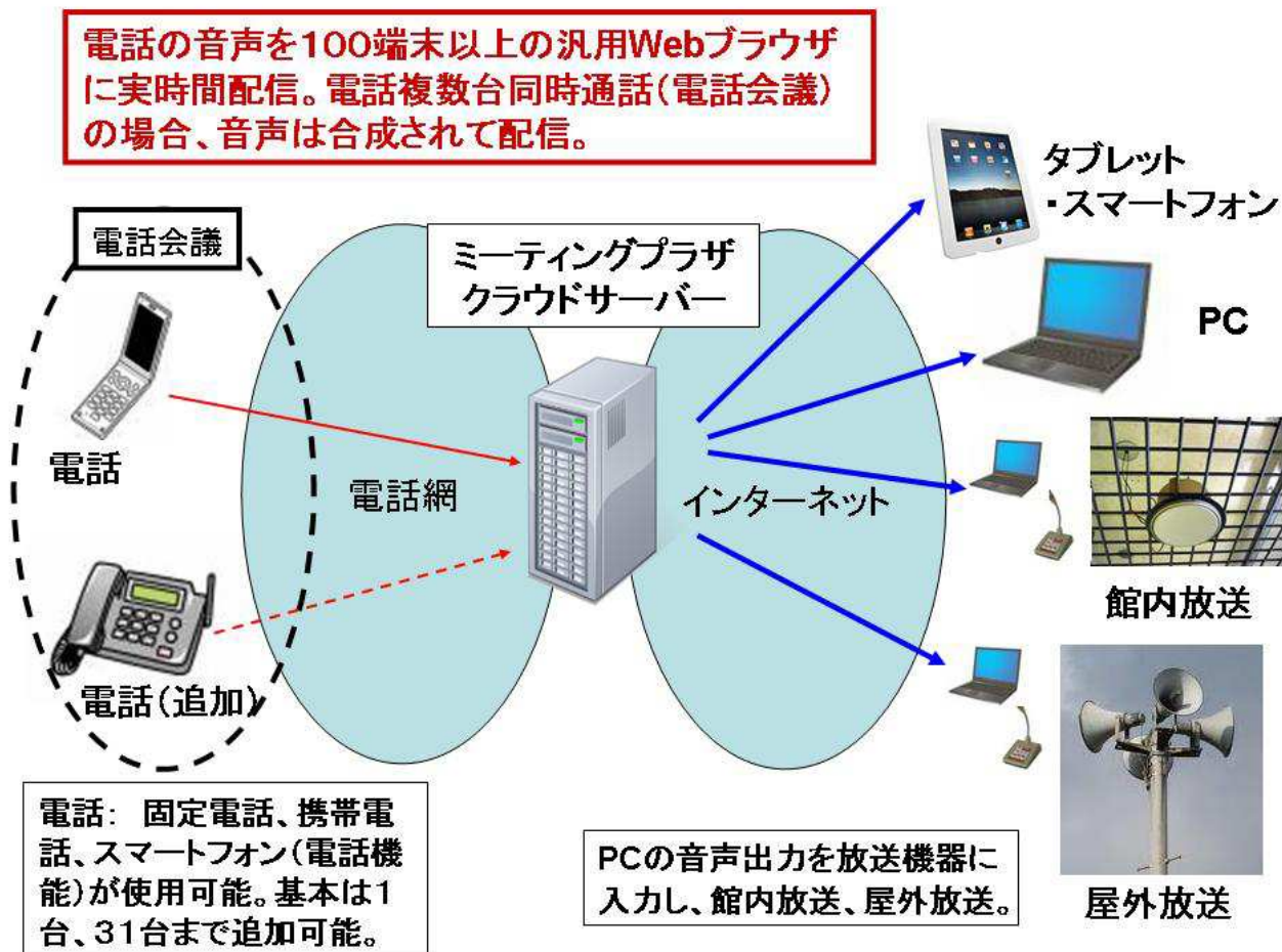
図1 ミーティングプラザ電話Web同報サービスの構成
