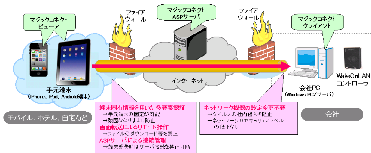
図1 「マジックコネクト・モバイル」クラウドサービスの構成
