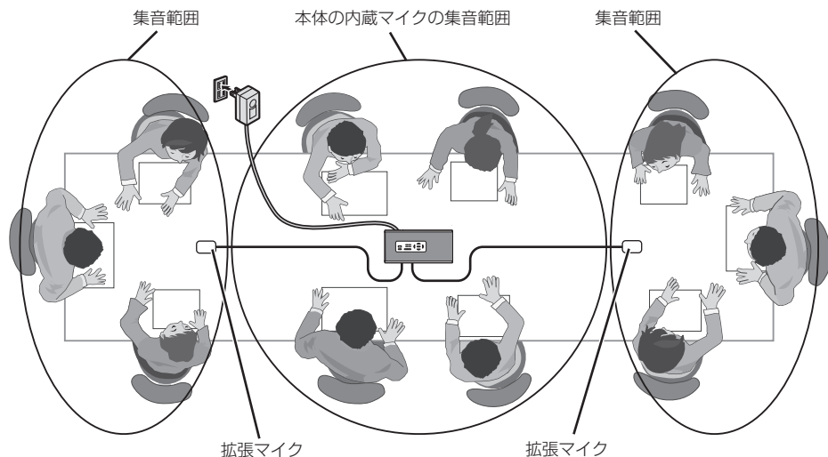
拡張マイク
