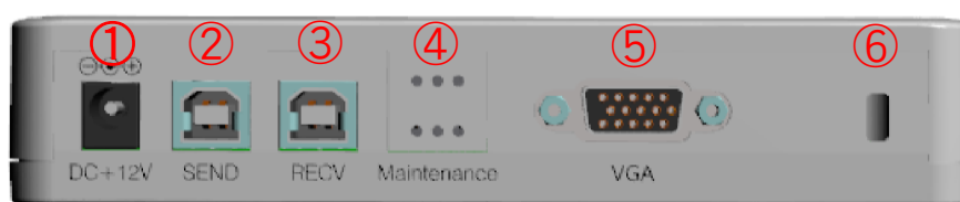
図 3-2 データブリッジ 背面
